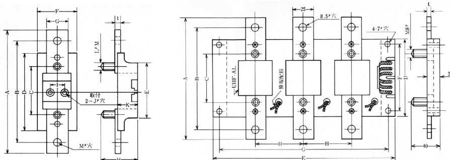
UHF-SB 1P寸法
