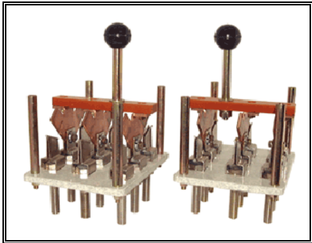
電源用スイッチ製作例①
