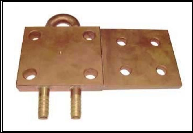
水冷ヒートシンク 製作例①
