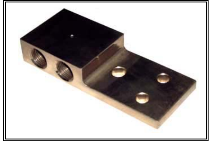
水冷ヒートシンク 製作例②
