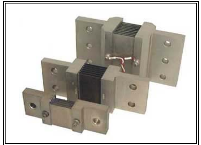
シャント 製作例
