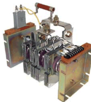
風冷スタック構成例
